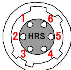
図 3-3-1 カメラ側電源コネクタ（ヒロセ：HR10G-7R-6PB）
