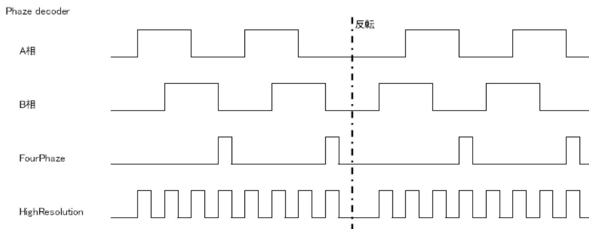
図 4-2-8-4-2 Encoder Mode
