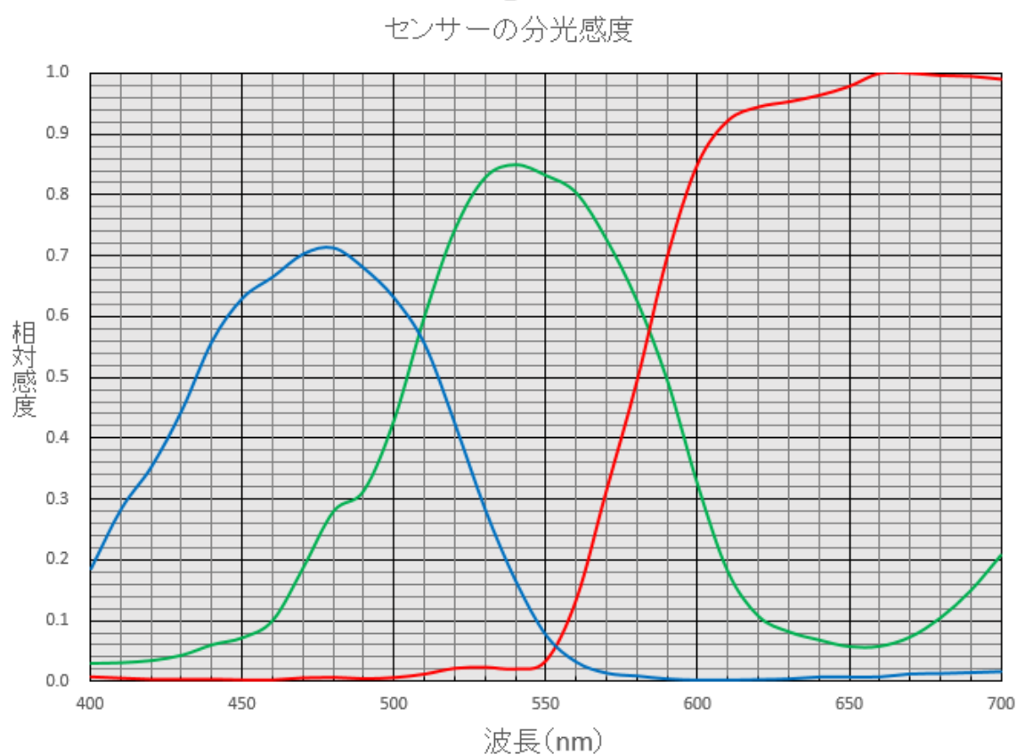
図 1-5-1 カメラ分光感度特性
