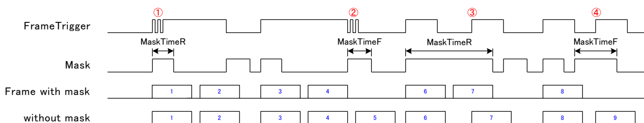
図 4-2-7-6 外部フレームトリガ入力とマスクの効果
