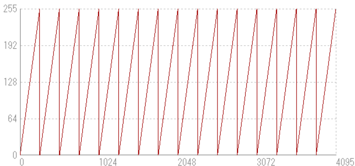
図 4-2-3-9(A) RCDL4K8GE GreyHorizontalRamp
