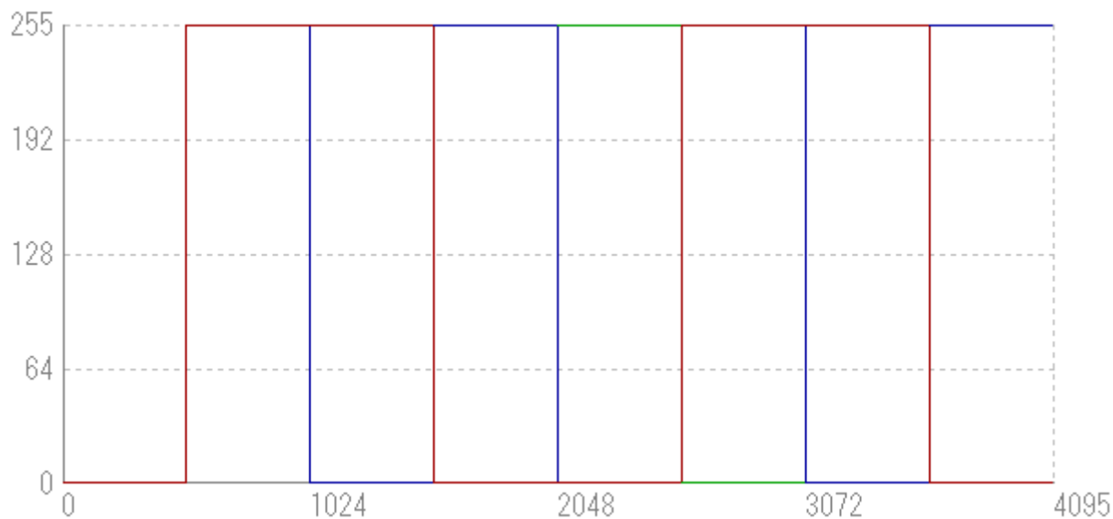
図 4-2-3-9(E) RC DL4K8GE Color Bar
