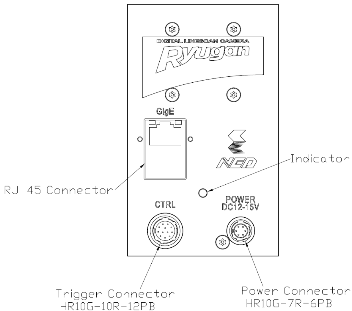
図 3-2-1 コネクタの配置 (RJ45 コネクタ、電源、外部トリガ、インディケータ)
