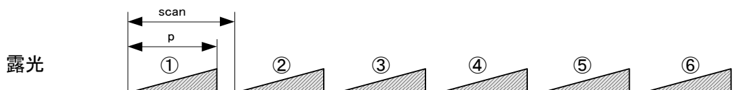
図 4-5-1-1 フリーラン露光モード
