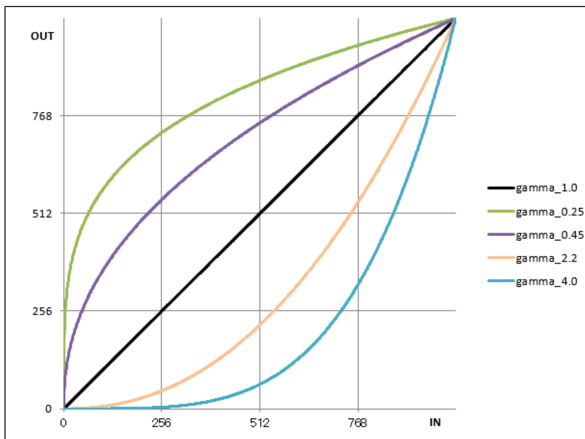
図 4-10-4 ガンマ補正特性
