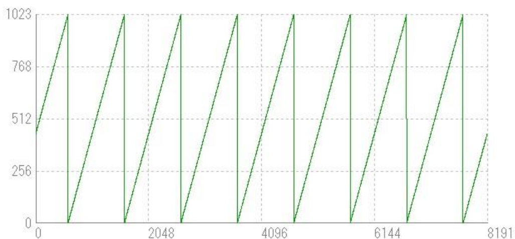
図 4-10-5-2-1 ライン1 Mono10 の NED_GreyDiagonalRamp 波形
