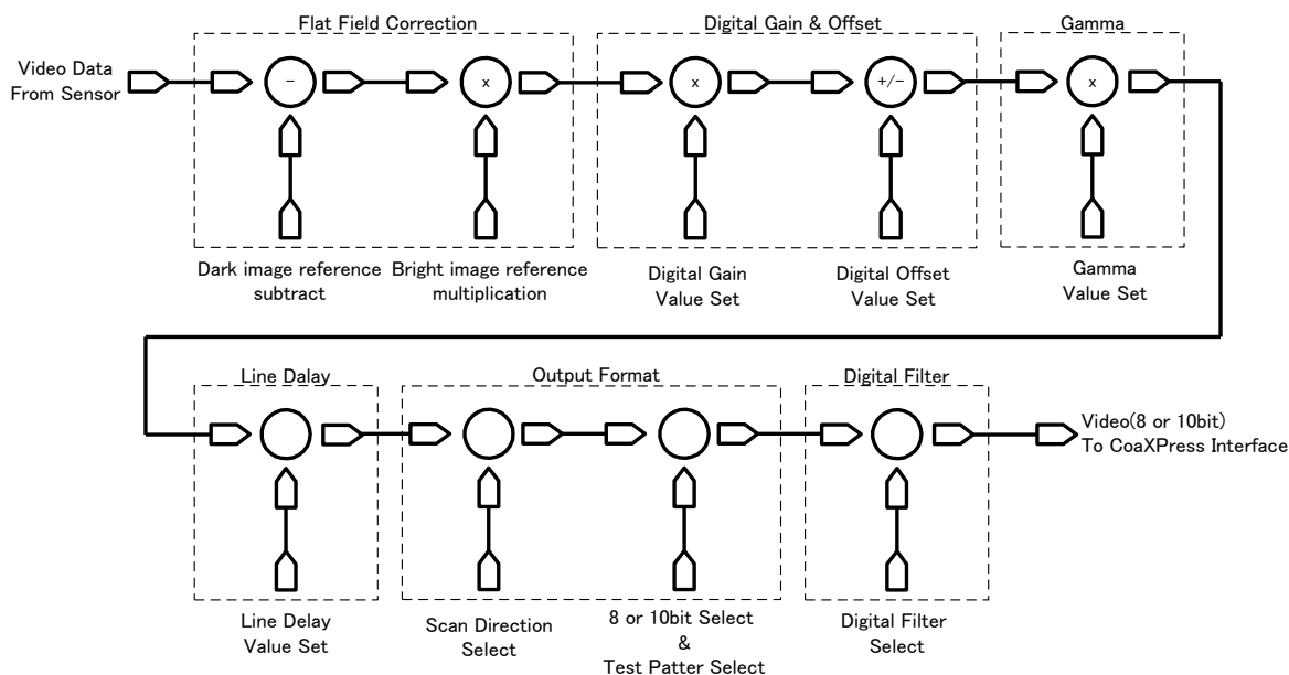
図 4-3-1 FPGA のプロセスブロックダイアグラム
