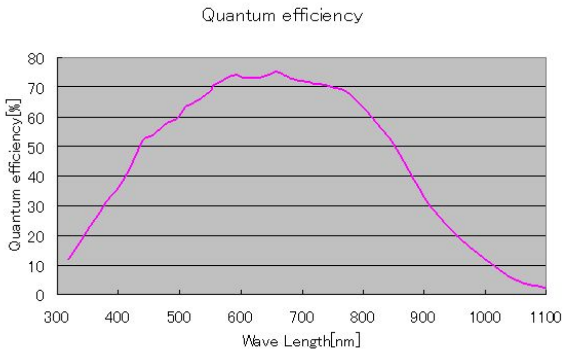
図 1-4-1 量子効率 (Max)
