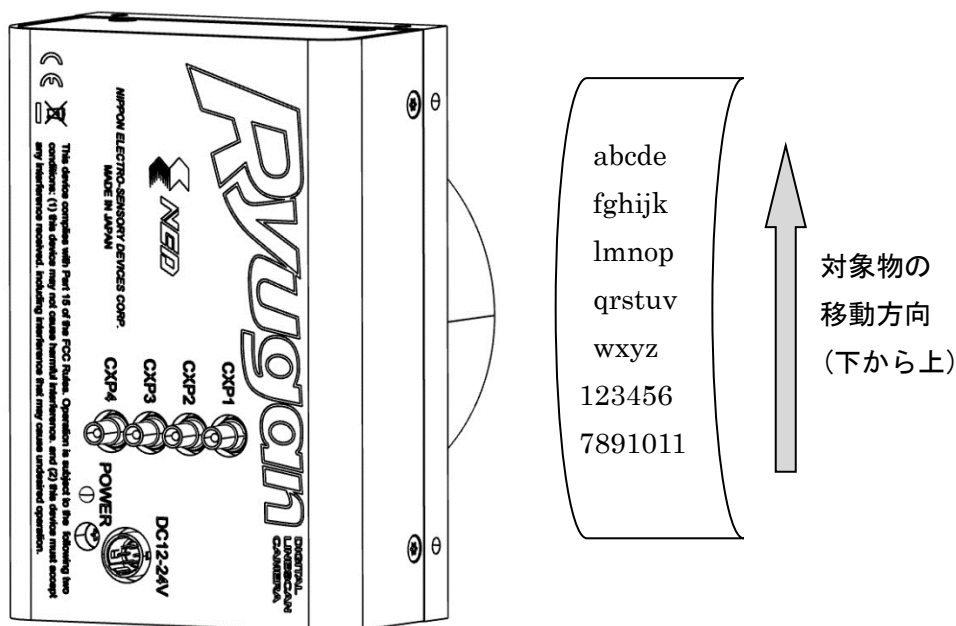
図 4-12-2 カメラの設置とラインディレイ ( NED_LineSpatialCorrection=1.0 の時)
