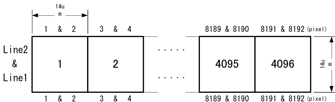
図 3-3-2 ビニングモード時のイメージ
