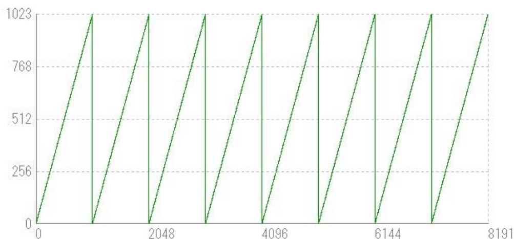
図 4-10-5-1-1 ライン1 Mono10 の GreyHorizontalRamp 波形
