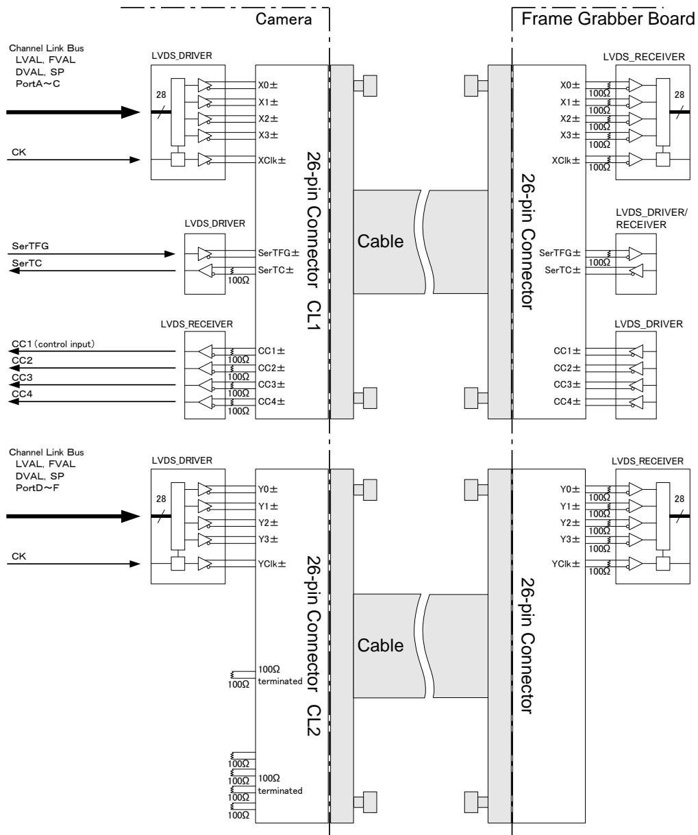
図 3-3-1 Camera/ Frame Grabber インターフェース (Base, Medium)
