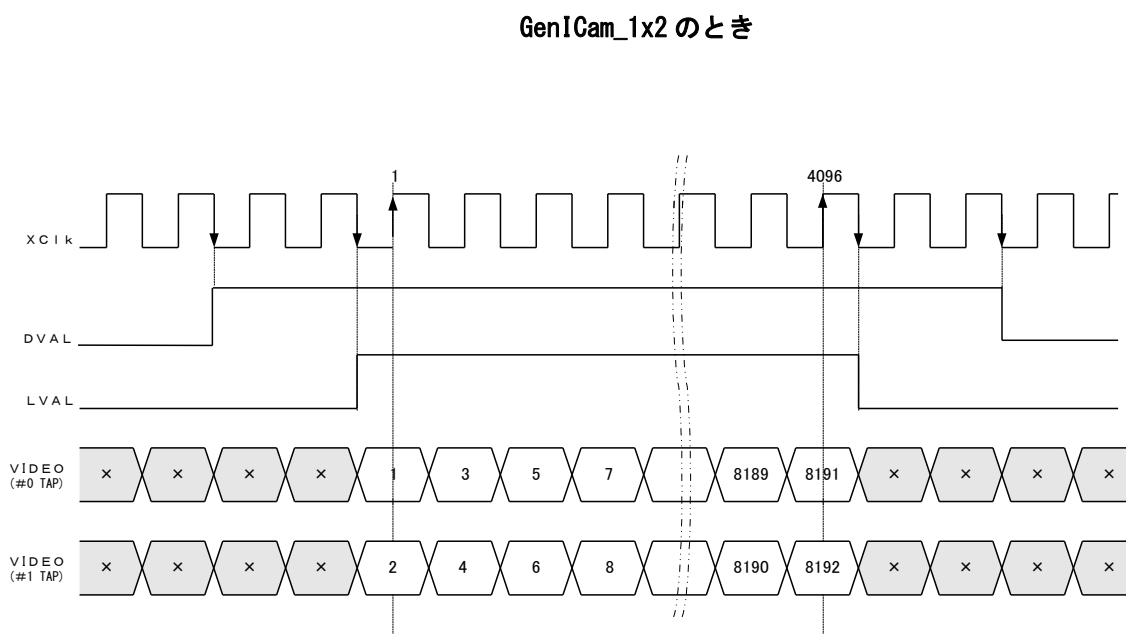
図 4-7-2a ビデオ出力位相関係
