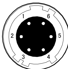
図 3-3-4 カメラ側電源コネクタ（ヒロセ：HR10G-7R-6PB）
